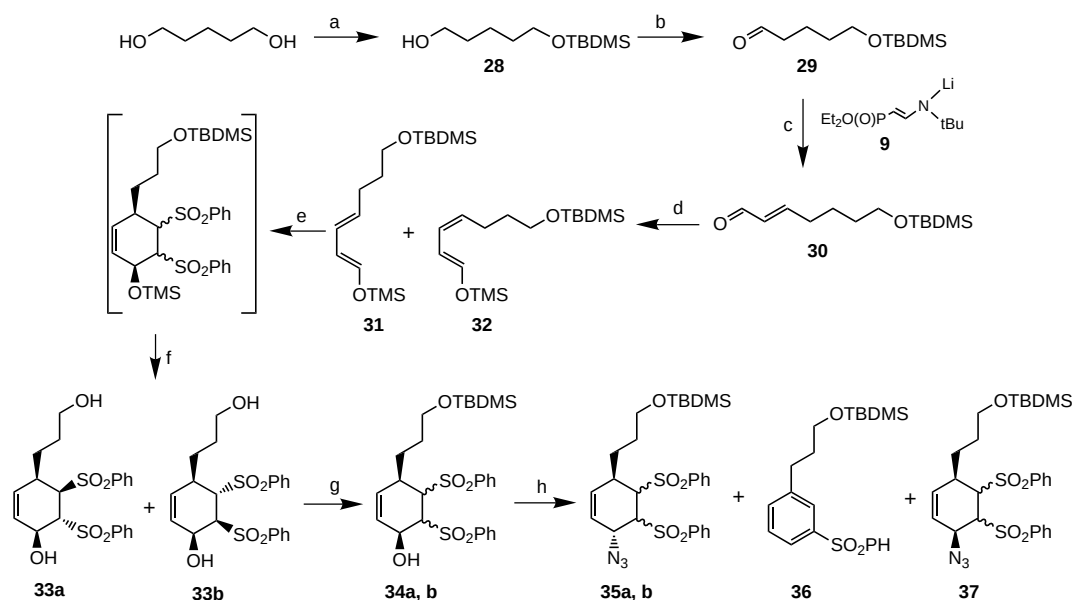
Scheme 9. a) NaH, TBDMSCl, THF, RT, 89%. b) (COCl) 2 , DMSO, CH 2 Cl 2 , -60 °C; NEt 3 , -20 °C, 90%. c) LDA, t BuN=CH-CH 3 , (EtO) 2 P(O)Cl, THF, -78 °C; H 3 O + , RT, 56%. d) TMSBr, ZnCl 2 , NEt 3 , toluene, reflux, 75%. e) 14 , ortho -xylene, 120 °C. f) MeOH, H + , RT, 66%. g) TBDMSCl, DMAP, CH 2 Cl 2 , NEt 3 , 83%. h) PPh 3 , DIAD, (PhO) 2 P(O)N 3 , CH 2 Cl 2 , 0 °C, 35a,b : 52%.
