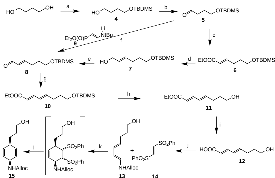
Scheme 4. a) NaH, TBDMSCl, THF, 97%. b) (COCl) 2 , DMSO, CH 2 Cl 2 , –60 °C; NEt 3 , –20 °C, 94%. c) NaH, (EtO) 2 P(O)CH 2 CO 2 Et, THF, –20 °C, 80%. d) DiBAH, CH 2 Cl 2 , –60 °C, 84%. e) (COCl) 2 , DMSO, CH 2 Cl 2 , –60 °C; NEt 3 , –20 °C, 94%. f) LDA, t BuN=CH–CH 3 , (EtO) 2 P(O)Cl, THF, –78 °C; H 3 O + , 67%. g) NaH, (EtO) 2 P(O)CH 2 CO 2 Et, THF, –20 °C, 70%. h) THF/H 2 O/CH 3 CO 2 H (1:1:3), 71%. i) NaOH, MeOH, 60 °C, 83%. j) (PhO) 2 P(O)N 3 , allyl alcohol, NEt 3 , reflux, 70%. k) 14 , ortho -xylene, reflux. l) Na(Hg), MeOH, KH 2 PO 4 , 37%.
